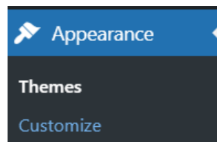
Slika 2. Podešavanja
