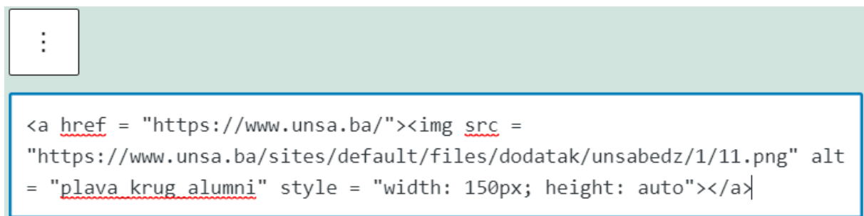
Slika 10. Kopiranje koda
