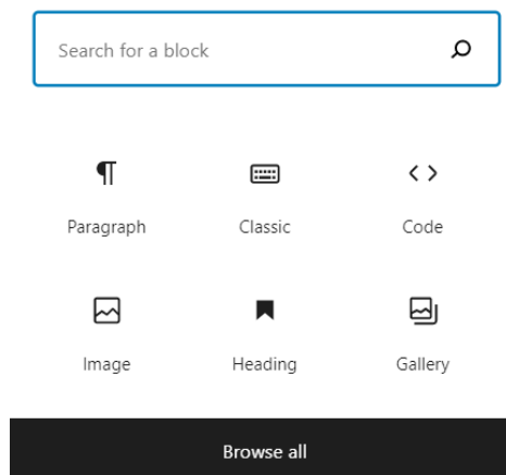
Slika 7. Odabir bloka
